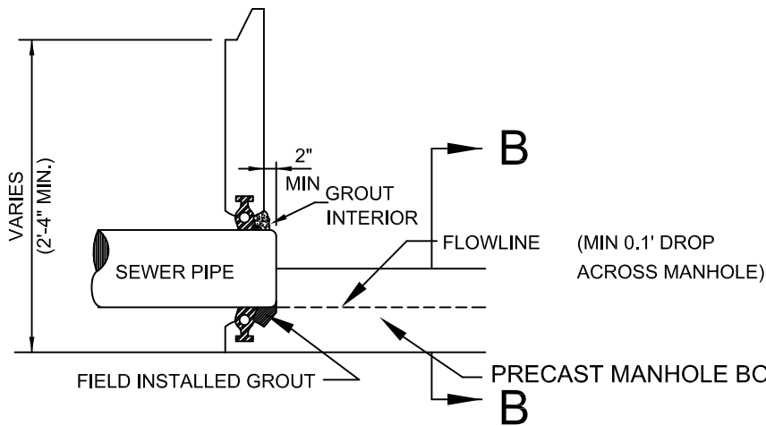
TYPE B MANHOLE
